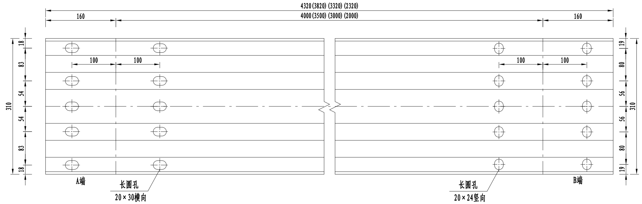
横梁C01平面图
