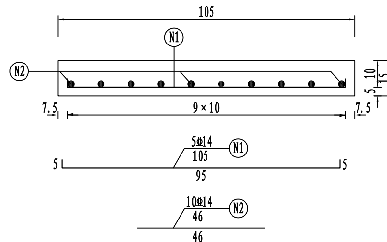
盖板立面
