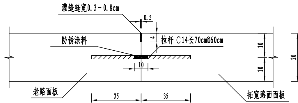
纵向施工缝结构大样图 (拼接加宽段) 1:10
