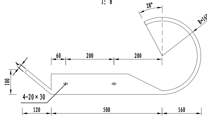
端头大样图
