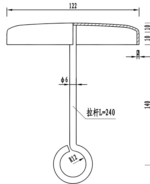
柱帽大样图
