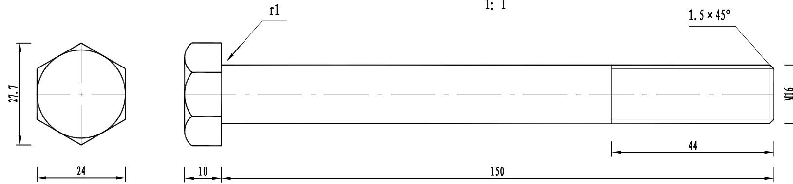
螺栓A大样图
