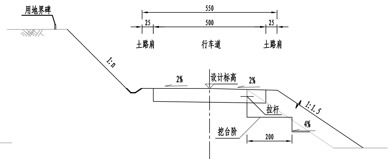
路基标准横断面图二 1:100
