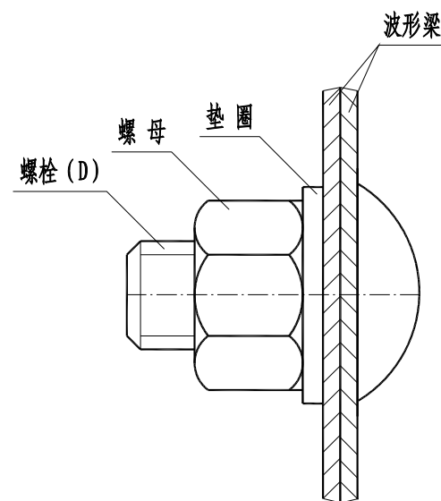
D节点大样图
