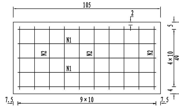
水沟盖板平面
