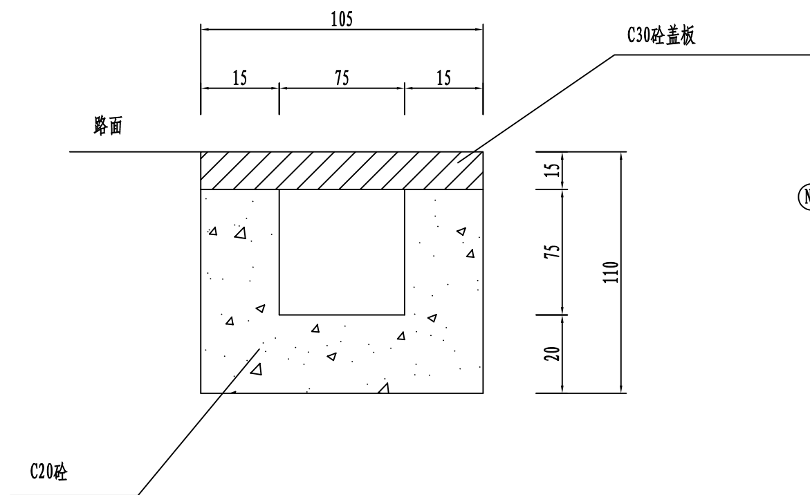
盖板沟 (1:50)
