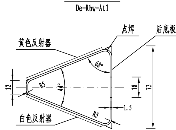
轮廓标平面图
