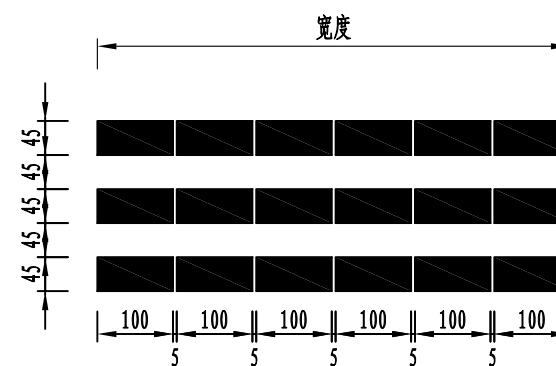
一组减速标线尺寸图
