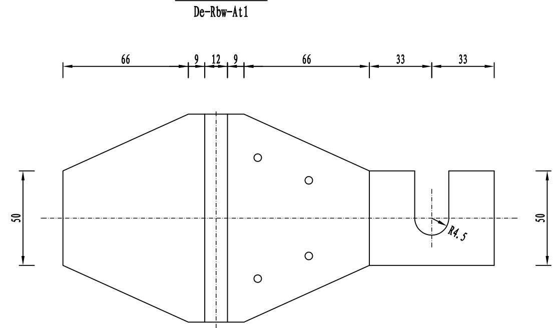
轮廓标展开图
